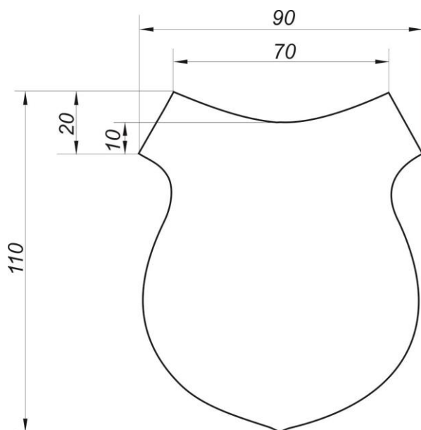
Rysunek nr. 7 - Taśma samoszczepna – pętelka do mocowania emblematu tarczy
