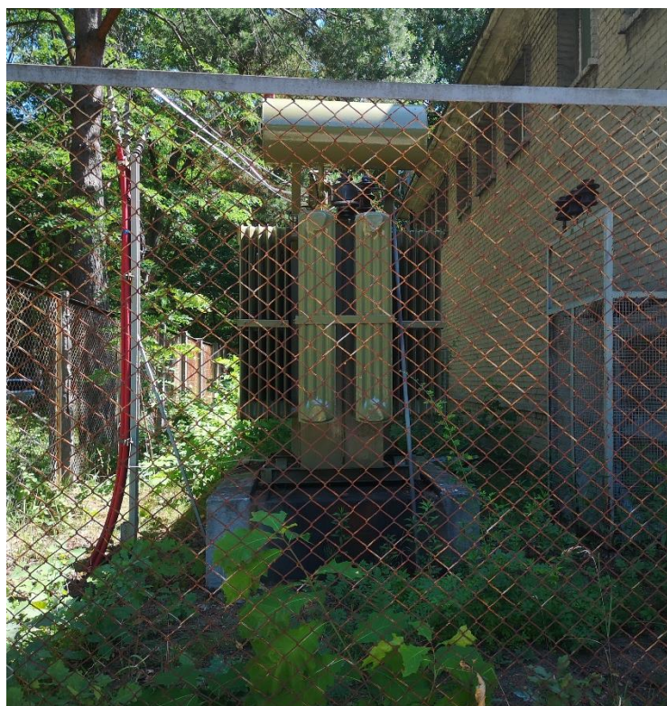
Fot. 6. Aktualny stan transformatora napowietrznego.
