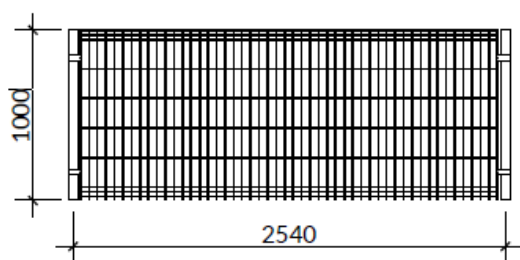
RZUT Z PRZODU (panel) SKALA 1:40
